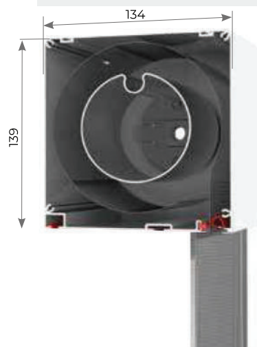
CASSONETTO 130
