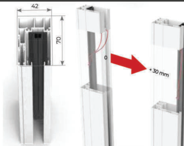
GUIDA MAGGIORATA +10% compensazione fino a 30 mm per lato
