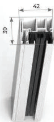
GUIDA STANDARD
