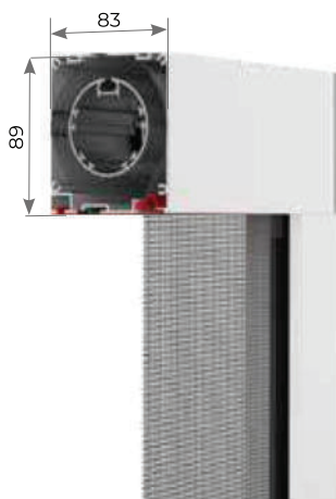
CASSONETTO 80
