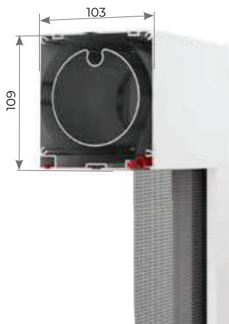
CASSONETTO 100
